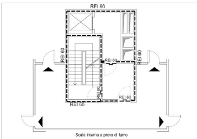
Scala a prova di fumo interna
