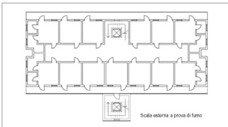
Scala a prova di fumo esterna
